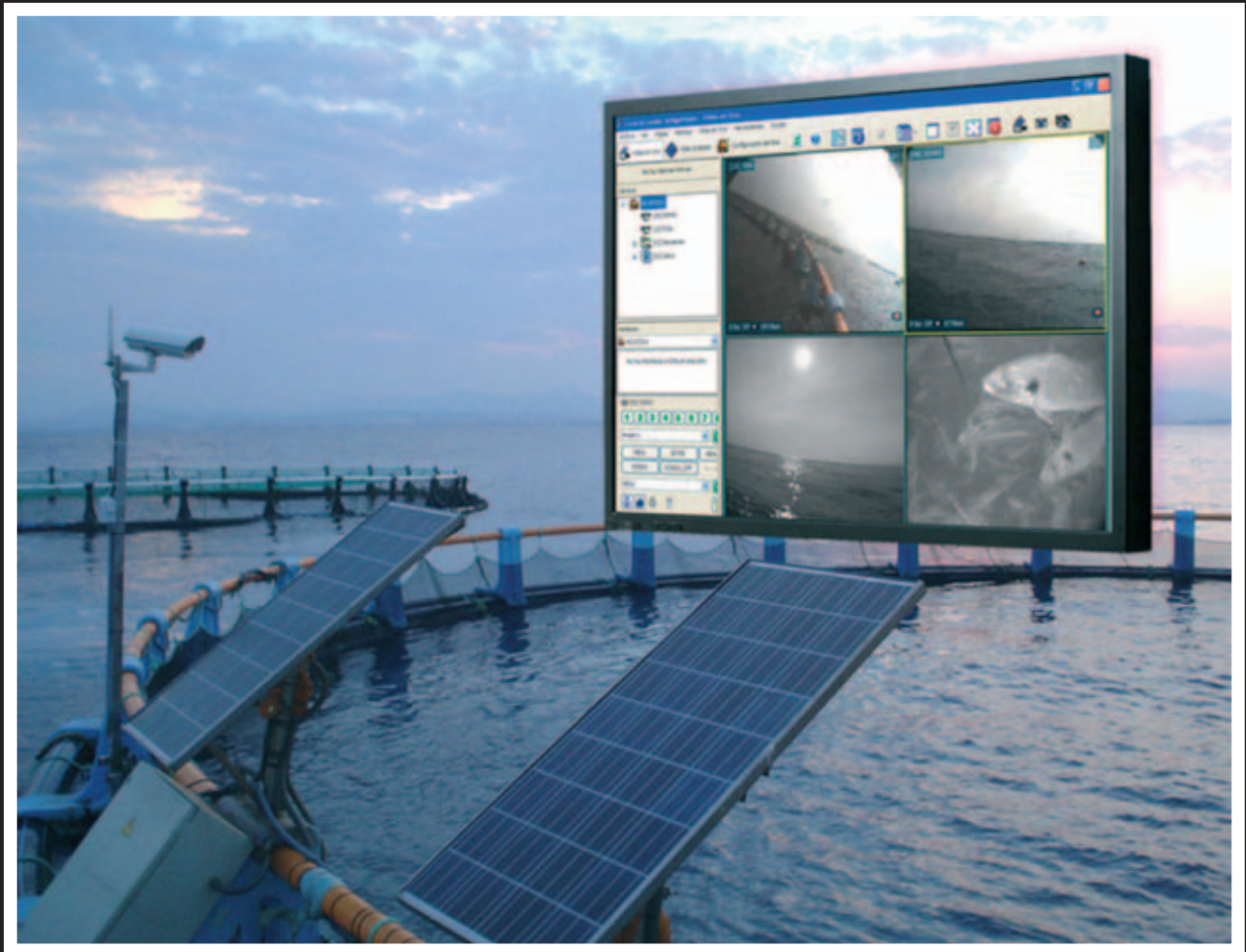
Vídeo por IP inalámbrico para la supervisión de una piscifactoría en alta mar.
